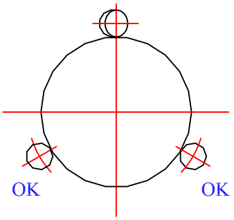
Alineacion caña luneta
